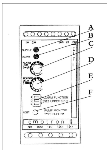
Obr. 6: Ovládací panel hlídače
