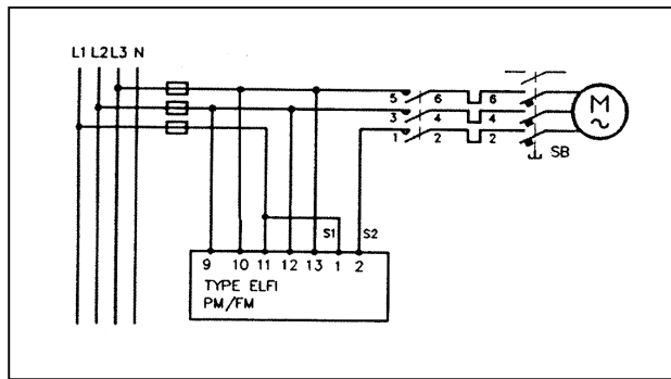
Obr. 4: Příklad přímého zapojení 3-fázového zdroje bez proudového transformátoru, to jest např. 3 x 400/400V max. 10 A. Jištění motoru je max. 20A - viz. technické údaje
