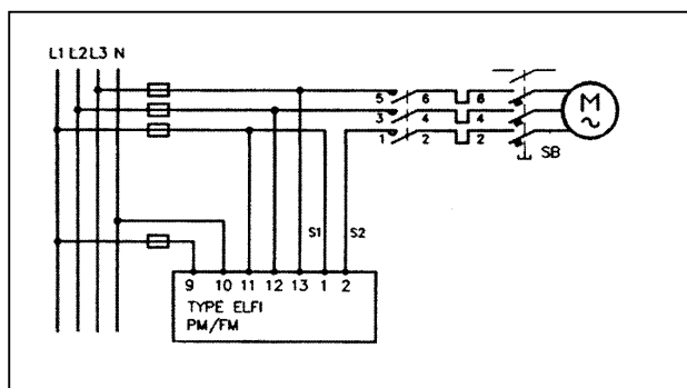
Obr. 2: Příklad zapojení bez proudového transformátoru. (jmenovitý proud motoru max. 10A)
