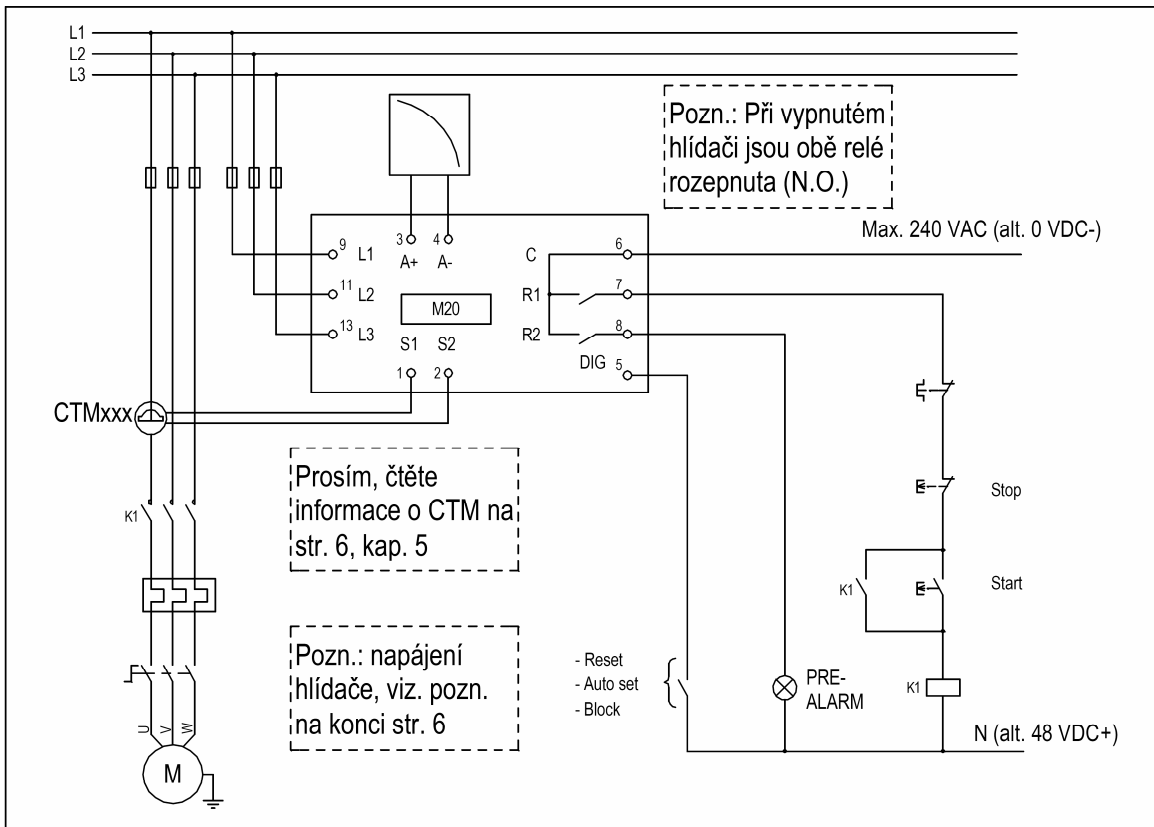
Obr. 1: Příklad zapojení
