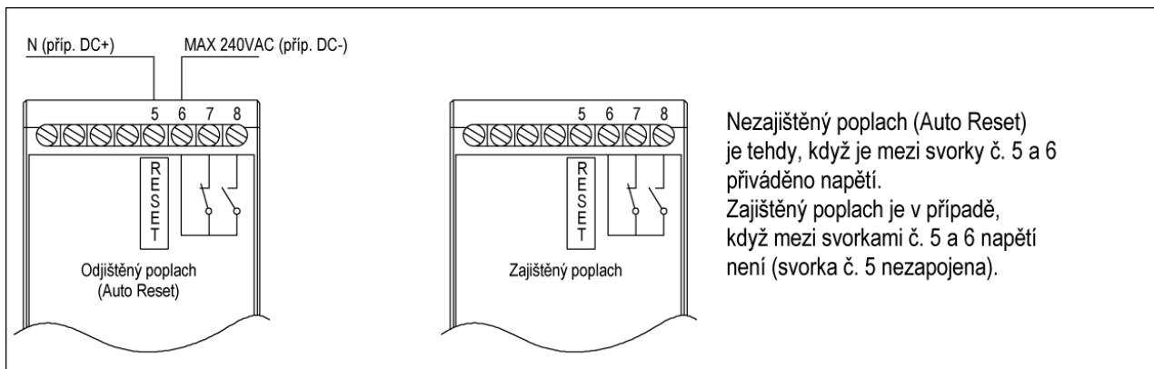
Obr. 3: Příklad zapojení zajištěného a odjištěného poplachu
