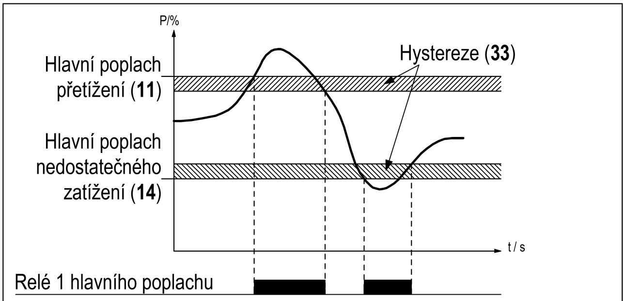
Obr. 10: Hystereze
