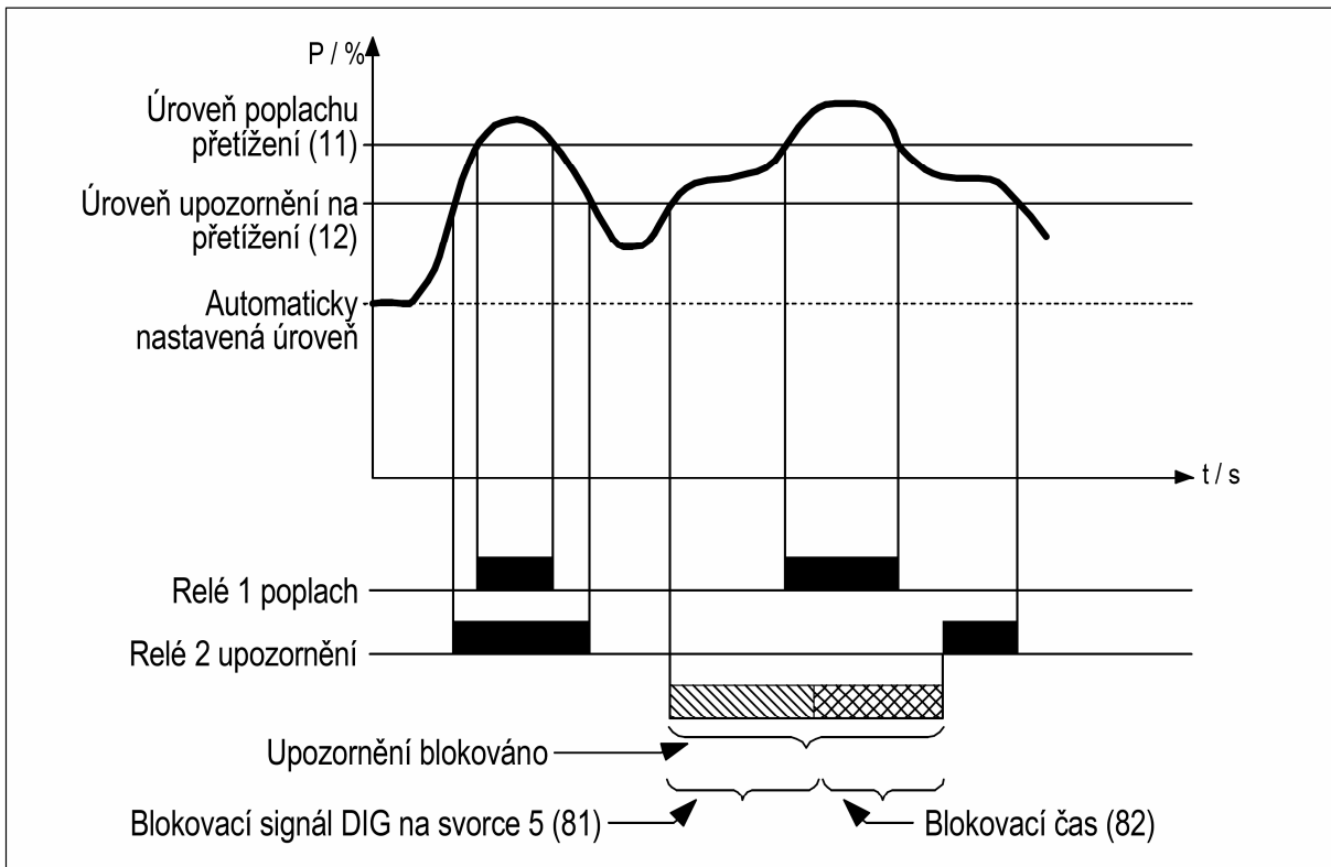
Obr. 11: Blokovací čas
