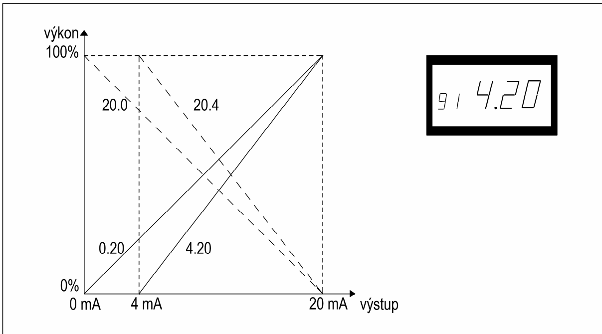
Obr. 12: Analogový výstup.
