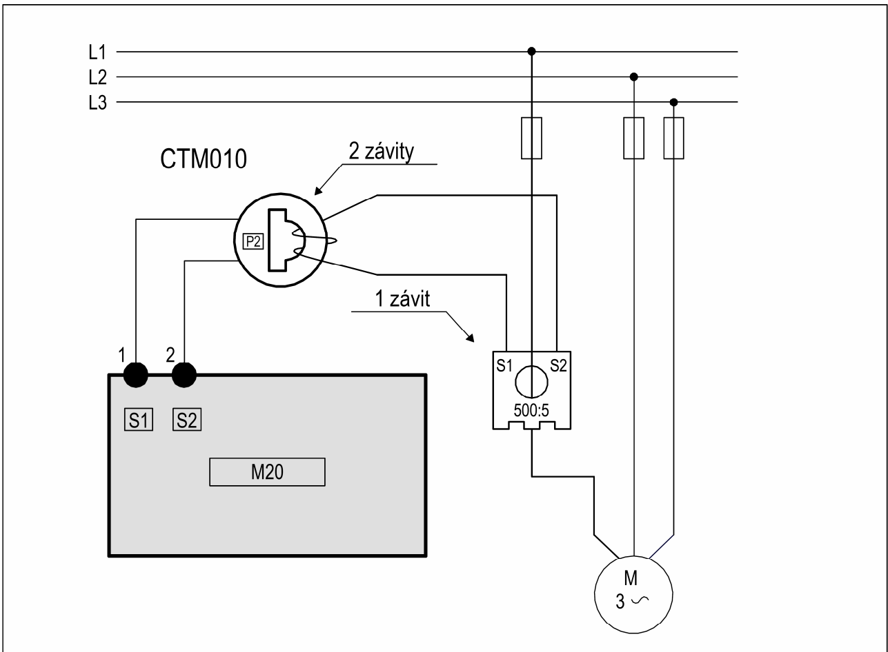
Obr. 6: Příklad zapojení CTM 010 se 2 závitů a primárním transformátorem 500:5 s 1 závitěm pro 260A motor.
