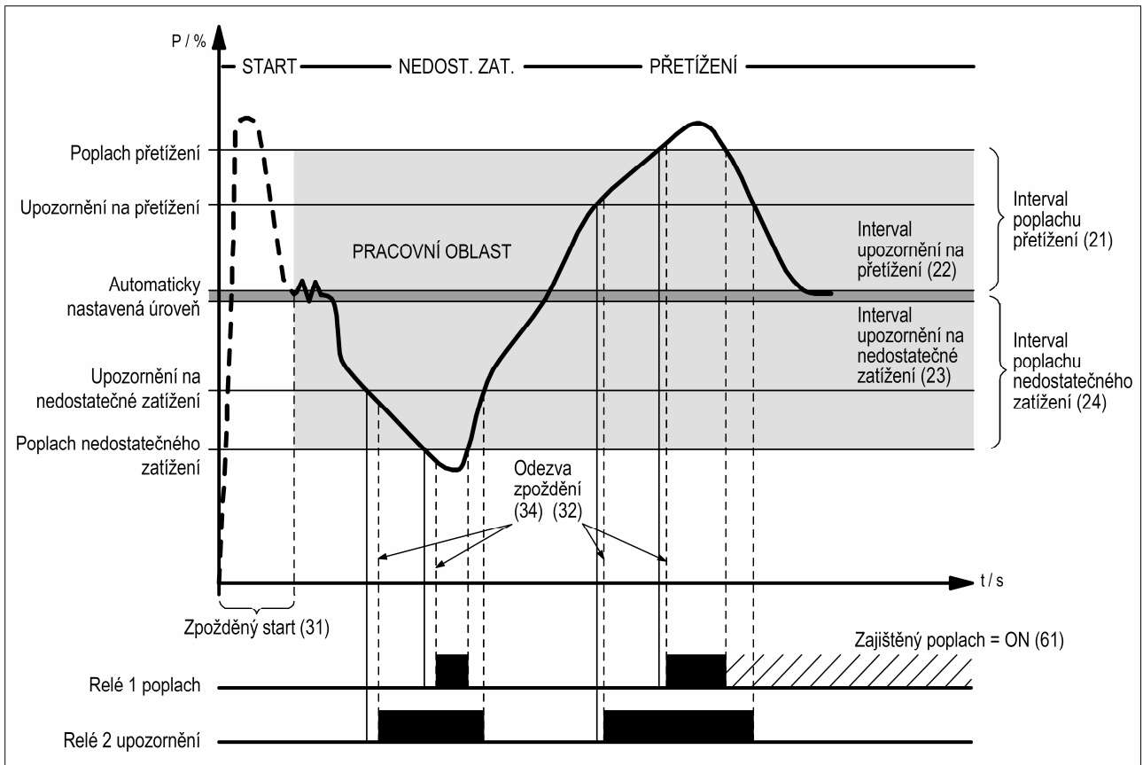
Obr. 7: Hlídač přetížení a nedostatečného zatížení
